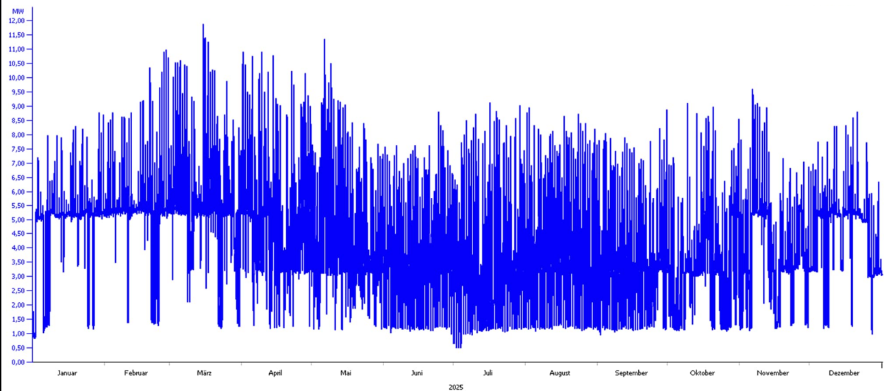
Summe aller Einspeisungen für Spannungsebene M und zeitlicher Verlauf
